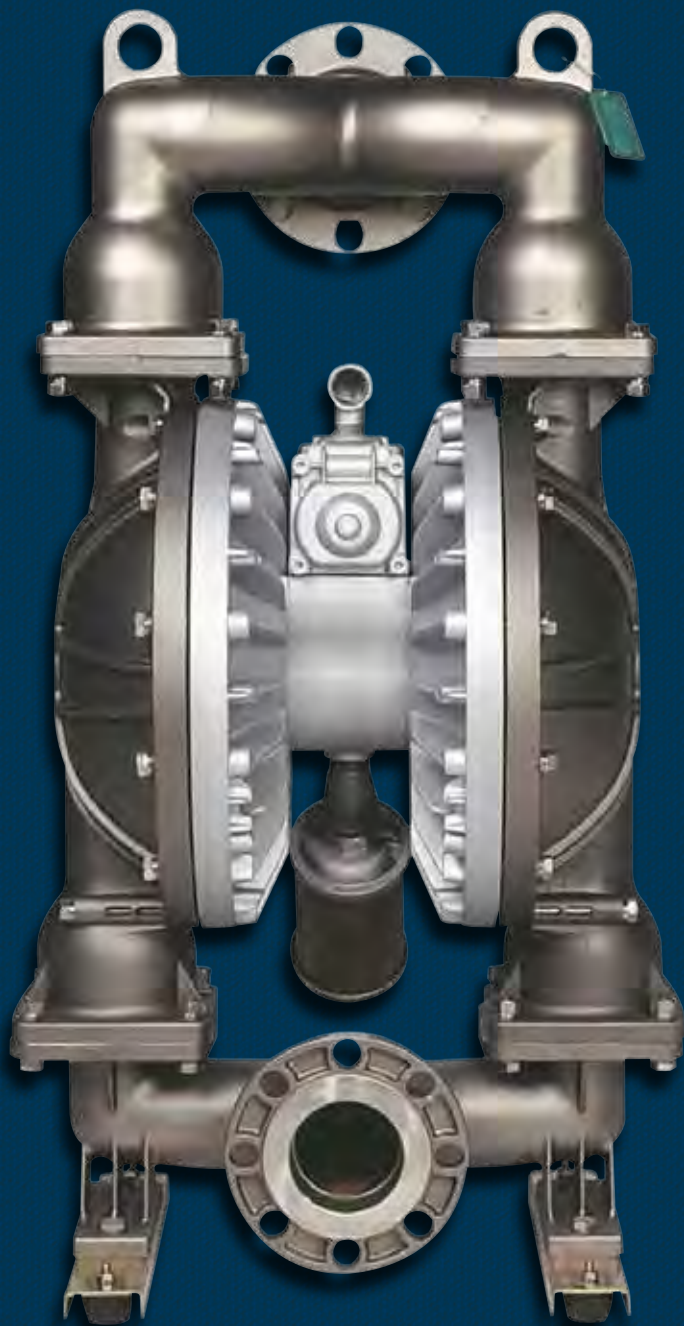
NDP-80 Алюминий Габариты: 522 мм x 998 мм Вес нетто: 62,0 кг Вес брутто: 77,0 кг
