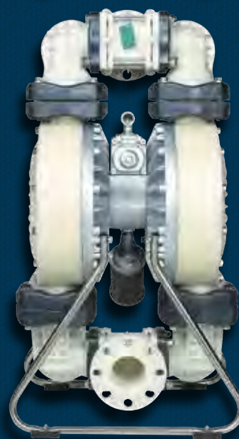
NDP-80 Полипропилен Габариты: 580 мм x 1044 мм Вес нетто: 70,0 кг Вес брутто: 85,0 кг
